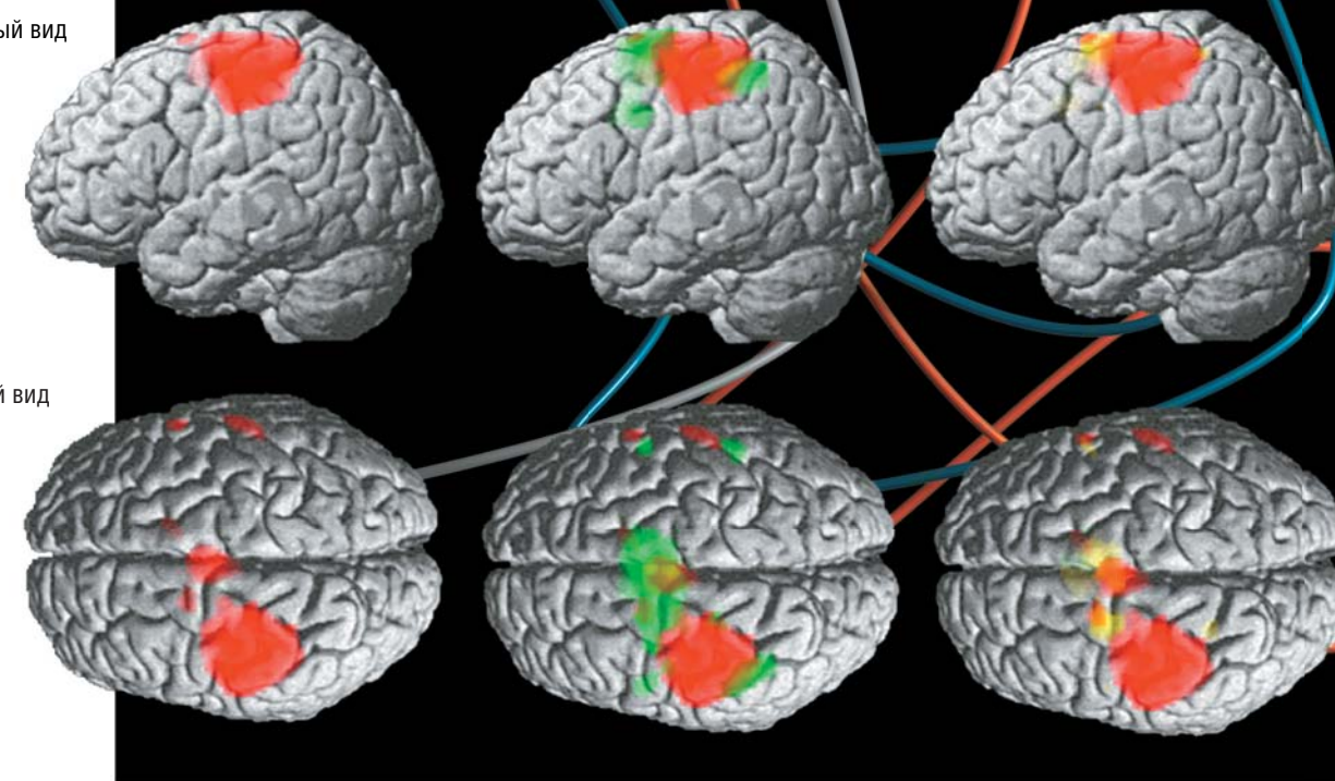
При реальном сжимании кисти в кулак происходит активация корковых моторных областей; аналогичный процесс идет и при попытке воспроизвести подобный ответ мозга усилием воли. В случае правой руки активируются участки в левой первичной моторной коре – целевом регионе (показаны красным цветом). Зеленым цветом отмечены области, активированные при нейробиоуправлении (приемы волевого управления по усмотрению пациента); желтым – области, активированные при попытках саморегуляции с помощью воображения действия. Видно, что в этом случае начинают работать соседние зоны мозга с небольшим перекрытием целевого региона. По: (Мельников и др., 2017)
